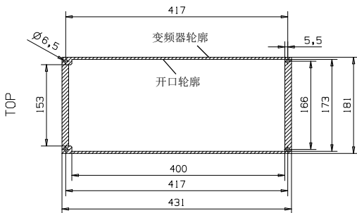
图 6: M15 法兰安装切断尺寸 (单位: mm)
