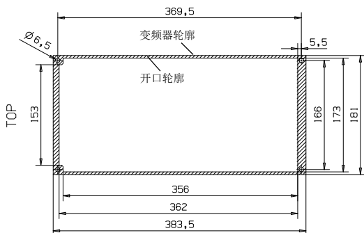
图 5: M14 法兰安装切断尺寸 (单位: mm)
