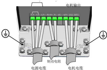
图 12: Vacon 20 M14 的电源连接
