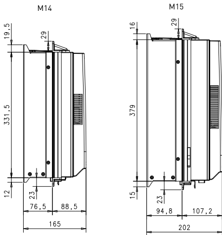
图 7: M14 和 M15 法兰安装深度尺寸 (单位: mm)
