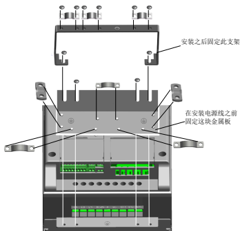
图 9: 附加 PE 板和 API 电缆支架, MI4 - MI5
