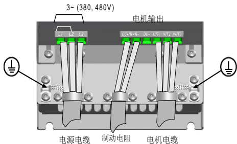
图 13: Vacon 20 M15 的电源连接
