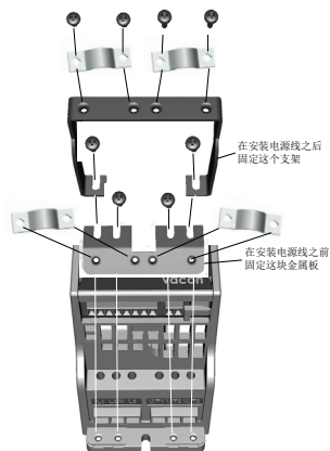
图 8: 附加 PE 板和 API 电缆支架, MI1 - MI3
